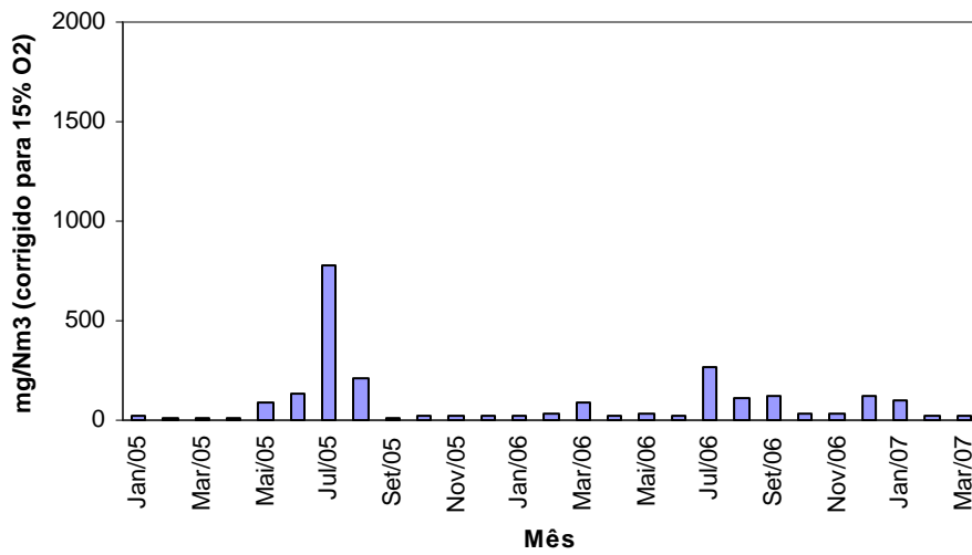
Gráfico n.º 4 - Carriço, SA - Cogeração - - Monóxido de Carbono Máximo Mensal das Médias Diárias
