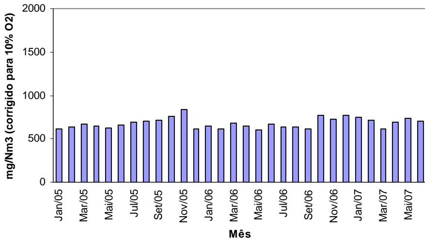
Gráfico n.º 33 - Cimpor (Souselas) - Forno 3 - Monóxido de Carbono Médias Mensais
