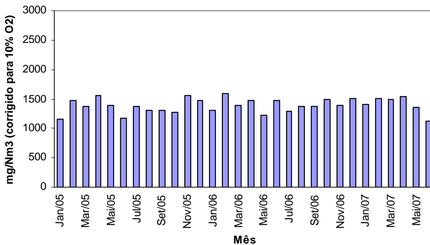
Gráfico n.º 19 - Cimpor (Souselas) - Forno 2 - Óxidos de Azoto Máximo Mensal das Médias Diárias
