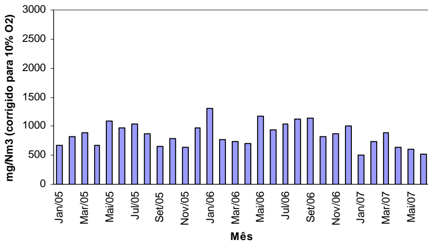
Gráfico n.º 32 - Cimpor (Souselas) - Forno 3 - Óxidos de Azoto Máximo Mensal das Médias Diárias
