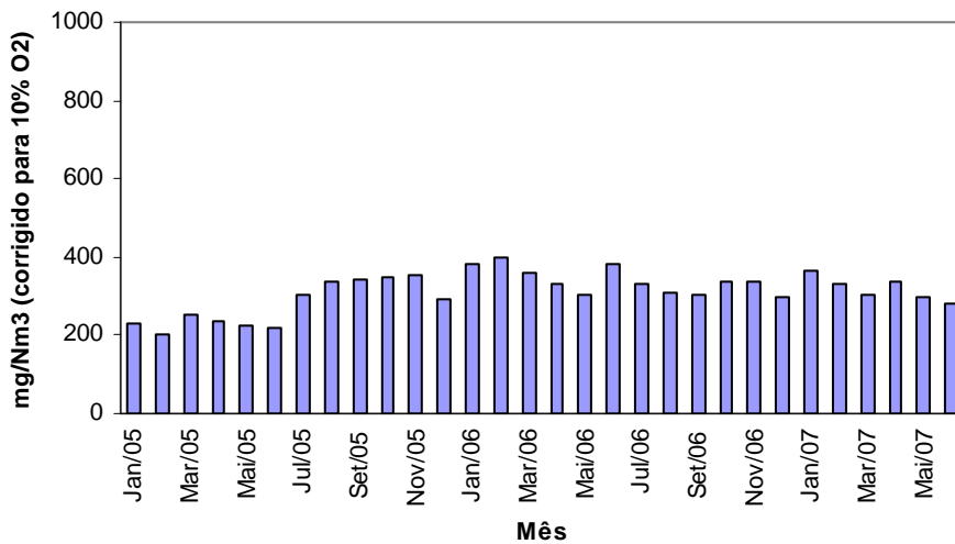
Gráfico n.º 30 - Cimpor (Souselas) - Forno 3 - Dióxido de Enxofre Máximo Mensal das Médias Diárias
