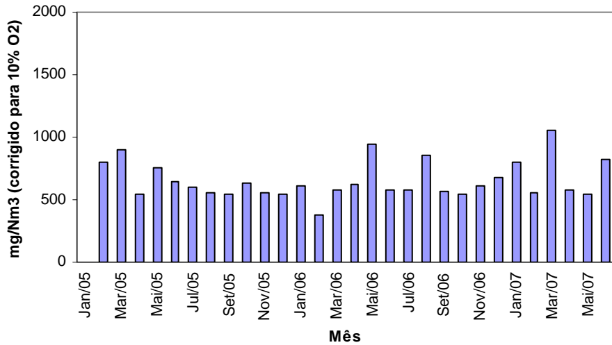
Gráfico n.º 8 - Cimpor (Souselas) - Forno 1 - Monóxido de Carbono Máximo Mensal das Médias Diárias
