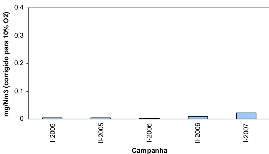
Gráfico n.º 25 - Cimpor (Souselas) - Forno 2 -Chumbo+Crómio+Cobre (Medição Pontual)
