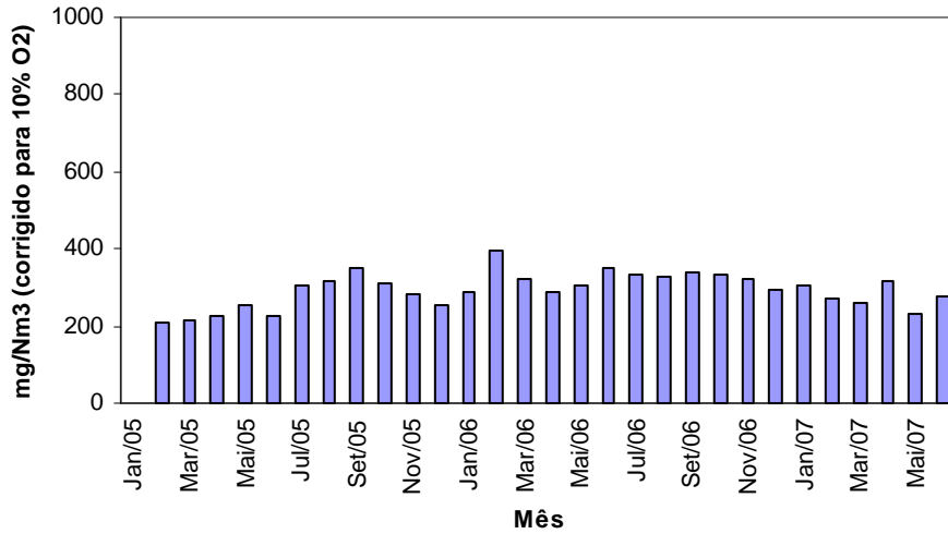
Gráfico n.º 3 - Cimpor (Souselas) - Forno 1 - Dióxido de Enxofre Médias Mensais
