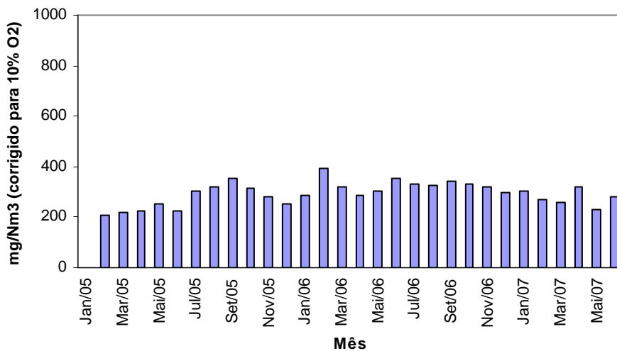
Gráfico n.º 4 - Cimpor (Souselas) - Forno 1 - Dióxido de Enxofre Máximo Mensal das Médias Diárias
