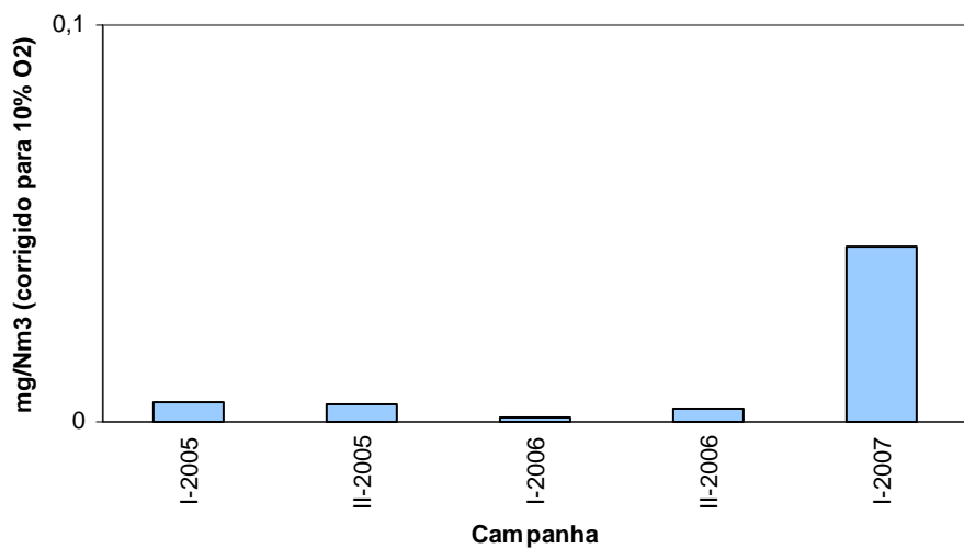
Gráfico n.º 24 - Cimpor (Souselas) - Forno 2 -Arsénio + Níquel (Medição Pontual)
