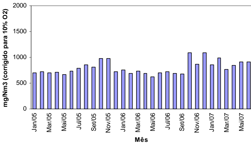
Gráfico n.º 34 - Cimpor (Souselas) - Forno 3 - Monóxido de Carbono Máximo Mensal das Médias Diárias
