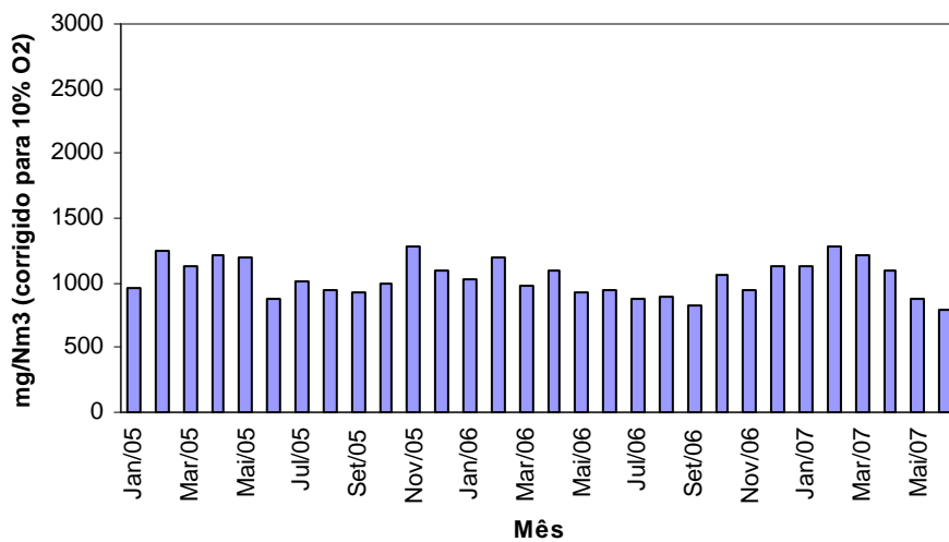
Gráfico n.º 18 - Cimpor (Souselas) - Forno 2 - Óxidos de Azoto Médias Mensais
