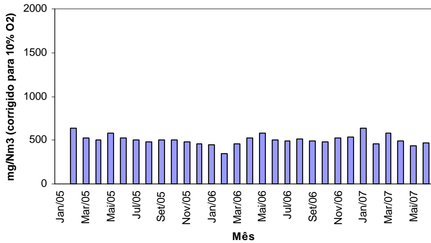
Gráfico n.º 7 - Cimpor (Souselas) - Forno 1 - Monóxido de Carbono Médias Mensais
