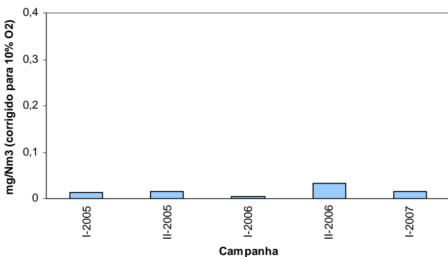
Gráfico n.º 12 - Cimpor (Souselas) - Forno 1 -Chumbo+Crómio+Cobre (Medição Pontual)
