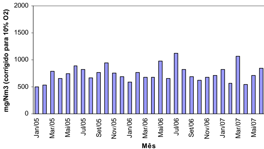
Gráfico n.º 21 - Cimpor (Souselas) - Forno 2 - Monóxido de Carbono Máximo Mensal das Médias Diárias
