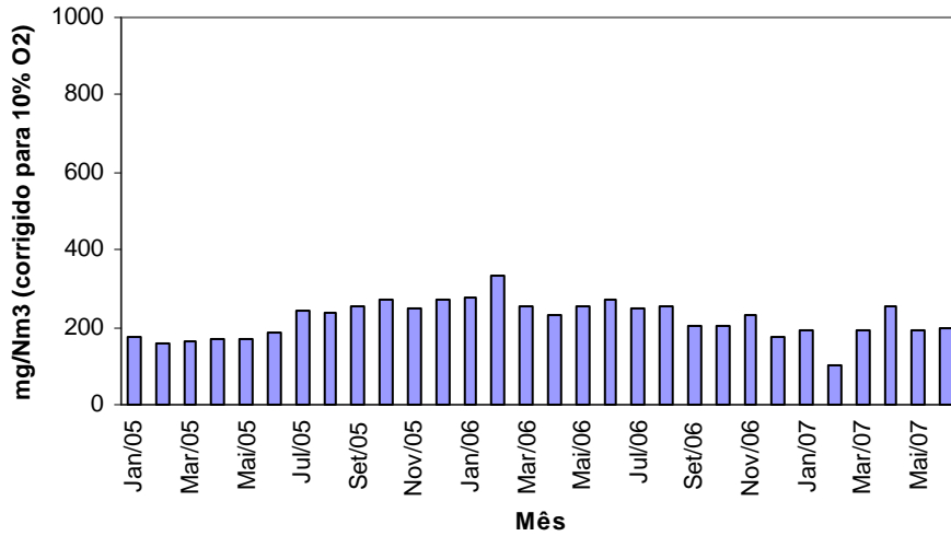
Gráfico n.º 16 - Cimpor (Souselas) - Forno 2 - Dióxido de Enxofre Médias Mensais
