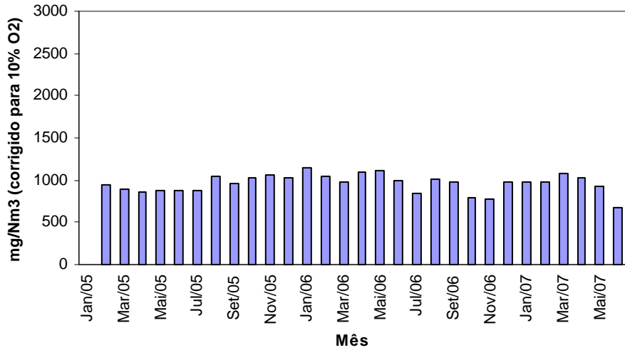
Gráfico n.º 5 - Cimpor (Souselas) - Forno 1 - Óxidos de Azoto Médias Mensais
