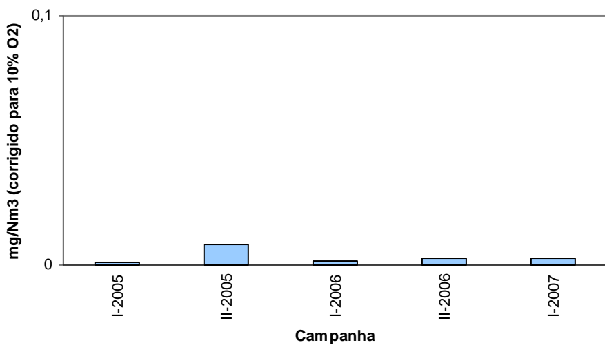
Gráfico n.º 11 - Cimpor (Souselas) - Forno 1 -Arsénio + Níquel (Medição Pontual)
