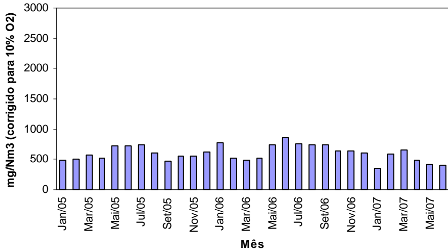
Gráfico n.º 31 - Cimpor (Souselas) - Forno 3 - Óxidos de Azoto Médias Mensais
