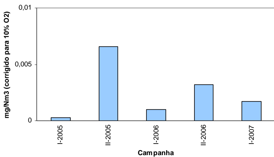
Gráfico n.º 37 - Cimpor (Souselas) - Forno 3 -Arsénio + Níquel (Medição Pontual)
