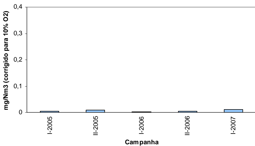
Gráfico n.º 38 - Cimpor (Souselas) - Forno 3 -Chumbo+Crómio+Cobre (Medição Pontual)
