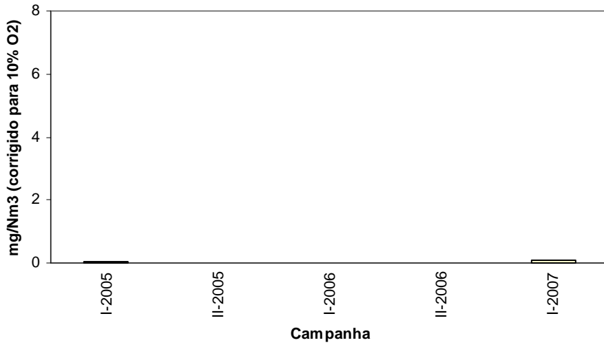
Gráfico n.º 26 - Cimpor (Souselas) - Forno 2 -Metais Pesados Totais (Medição Pontual)
