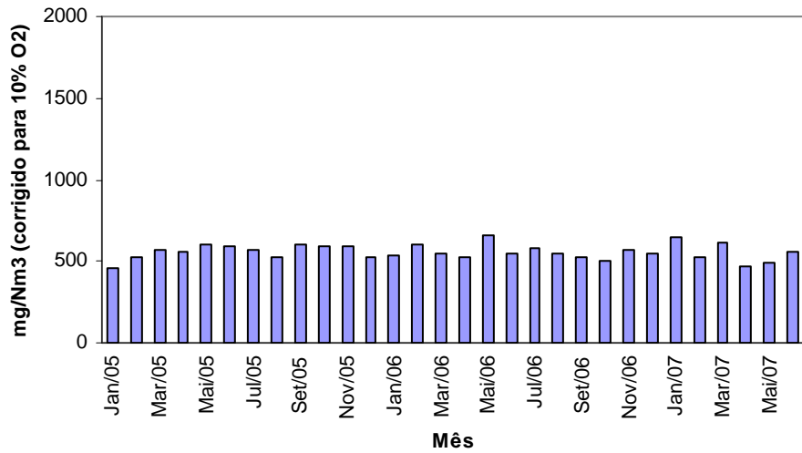
Gráfico n.º 20 - Cimpor (Souselas) - Forno 2 - Monóxido de Carbono Médias Mensais
