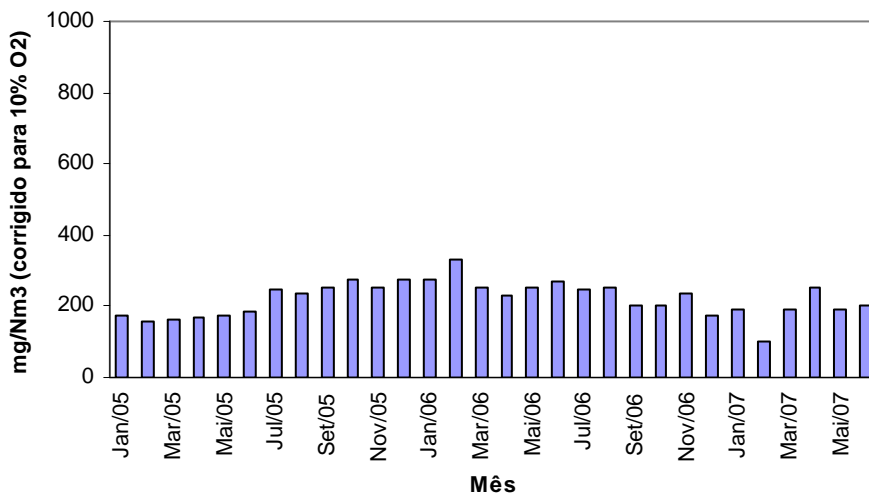
Gráfico n.º 17 - Cimpor (Souselas) - Forno 2 - Dióxido de Enxofre Máximo Mensal das Médias Diárias
