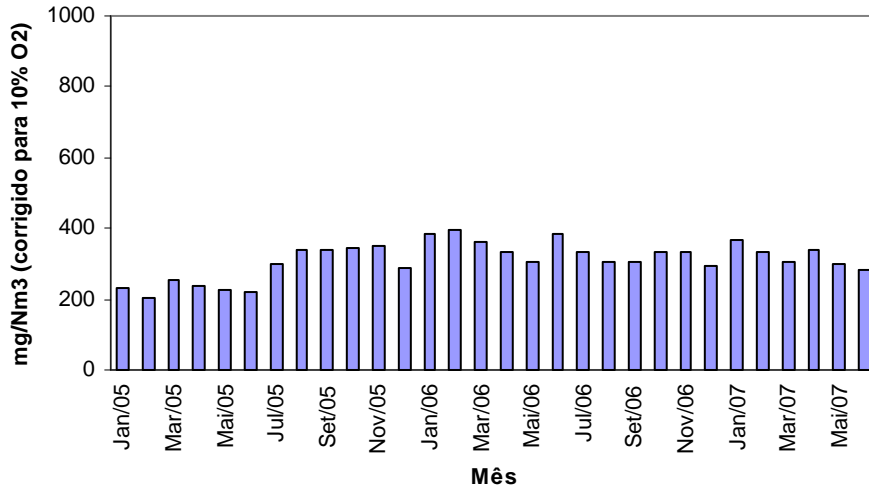
Gráfico n.º 29 - Cimpor (Souselas) - Forno 3 - Dióxido de Enxofre Médias Mensais
