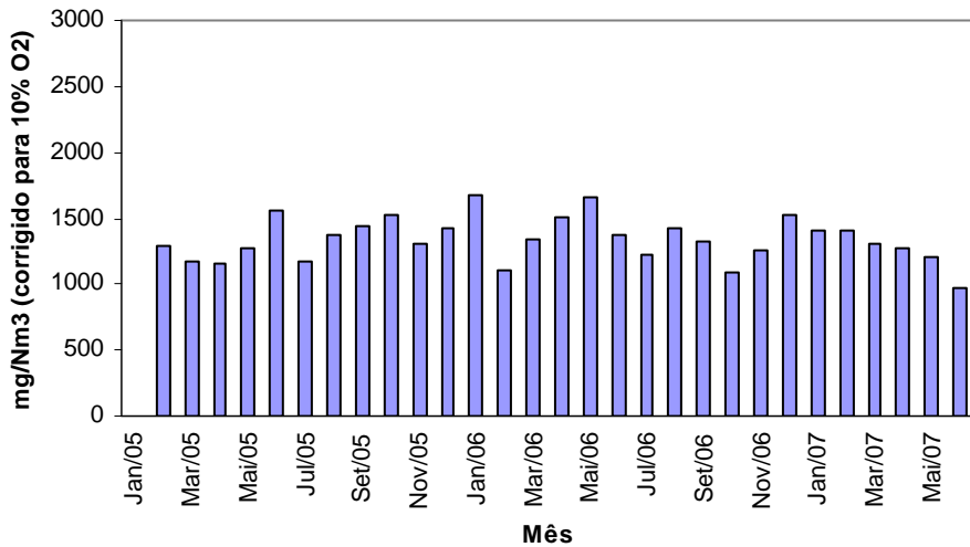
Gráfico n.º 6 - Cimpor (Souselas) - Forno 1 - Óxidos de Azoto Máximo Mensal das Médias Diárias
