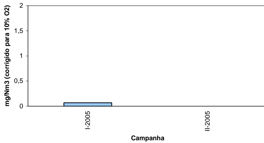
Gráfico n.º 21 - CMP (Maceira) - Forno 6 - Chumbo+Crómio+Cobre (Medição Pontual)
