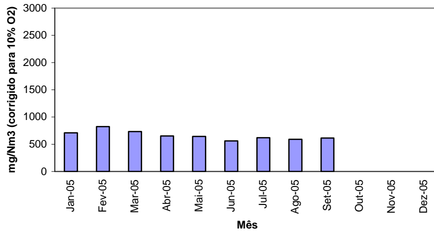
Gráfico n.º 17 - CMP (Maceira) - Forno 6 - Óxidos de Azoto Máximo Mensal das Médias Diárias
